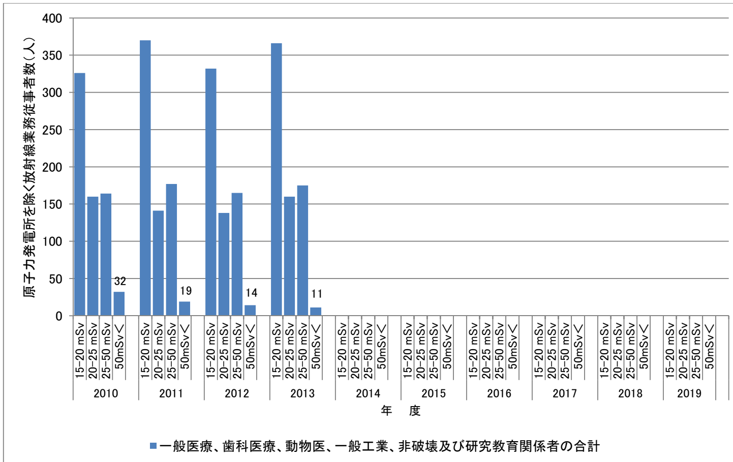
年間 15 mSv を超える原子力施設を除く放射線業務従事者の線量分布の年度推移(2010～2013)
