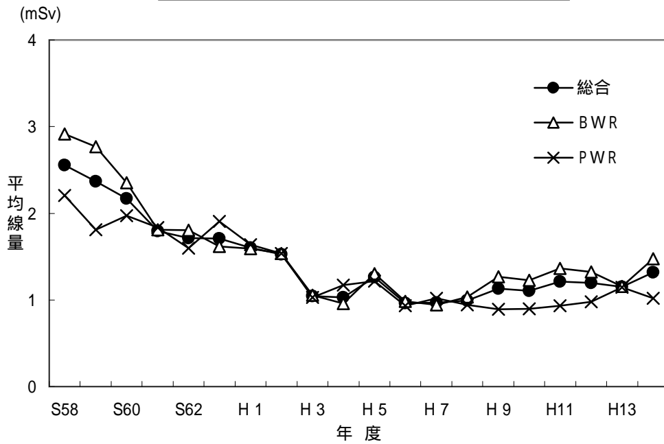
実用発電用原子炉施設における平均線量の年度別推移
